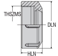
ER 25, 32, 40, 50
